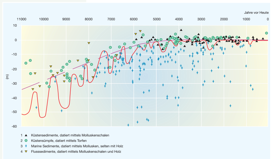
Unten: Die rote Kurve zeigt die mögliche Meeresspiegelentwicklung des Schwarzen Meeres für die letzten 11.000 Jahre (nach der Interpretation von Balabanov 2007). Zu erkennen sind starke Schwankungen zwischen Meeresspiegelanstieg (Transgression) und Meeresspiegelabfall (Regression). Die grüne Linie ist eine andere Interpretation der vorhandenen Daten.
