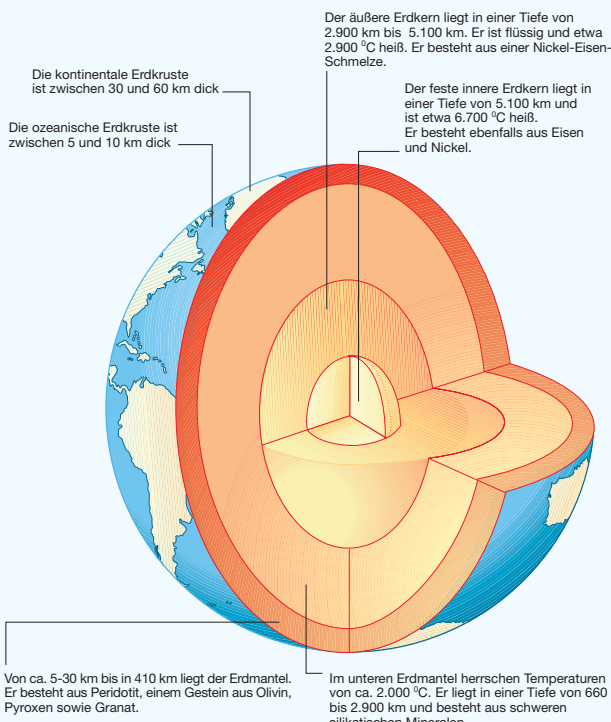
Oben: Die Abbildung zeigt den generellen Aufbau der Erde.
