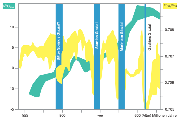
Oben: Weltweit wurden in Meeresablagerungen, die vor etwa 900-550 Mio. Jahren entstanden sind, die Isotopenverhältnisse von Strontium ( ^{87}\text{Sr}/^{86}\text{Sr} ) und Kohlenstoff ( \delta^{13}\text{C} ) gemessen. Die blau markierten Bereiche stellen Zeiten globaler Vereisungen dar.
